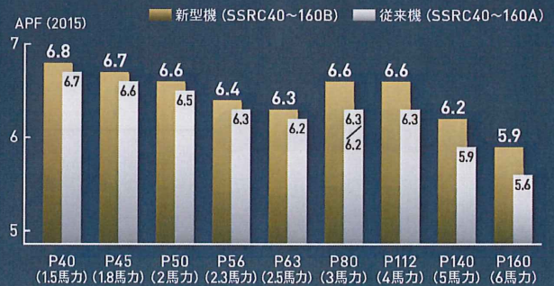
能力別APF(2015)値 APF値はJRA4002:2013Rに基づく。 【天井埋込カセット形エコ・ラウンドフロー (センシング) タイプ】
